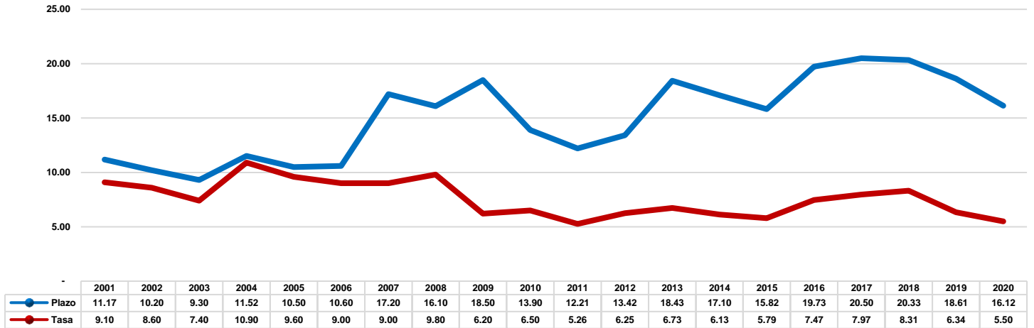
Gráfica No. 8. Comparativo del plazo promedio de vencimiento y la tasa de interés del financiamiento público del Estado de Nuevo León, 2001-2020. (Número de años y %).
