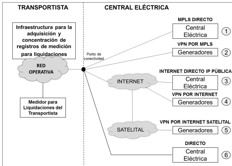
Figura 6.1 – Esquema del sistema de comunicaciones para la medición para liquidaciones, desde la Central Eléctrica hacia el Transportista
