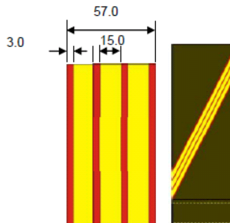
Acotación en milímetros
