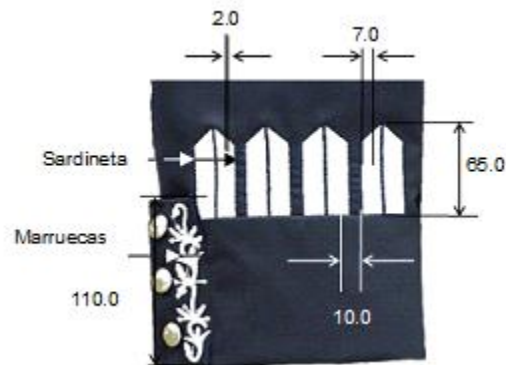
Acotaciones en milímetros
