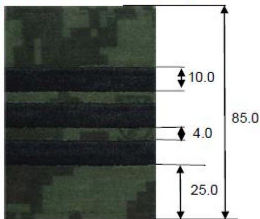
Acotación en milímetros
